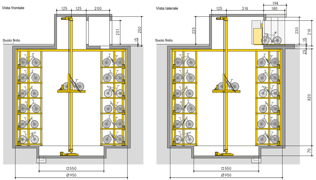
Sezione livello di parcheggio
